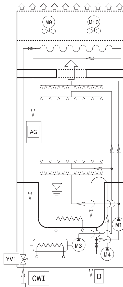
Diagram over hydrauliske kredsløb for automatisk hætteopvaskemaskine med energigenvinding (ESD)
