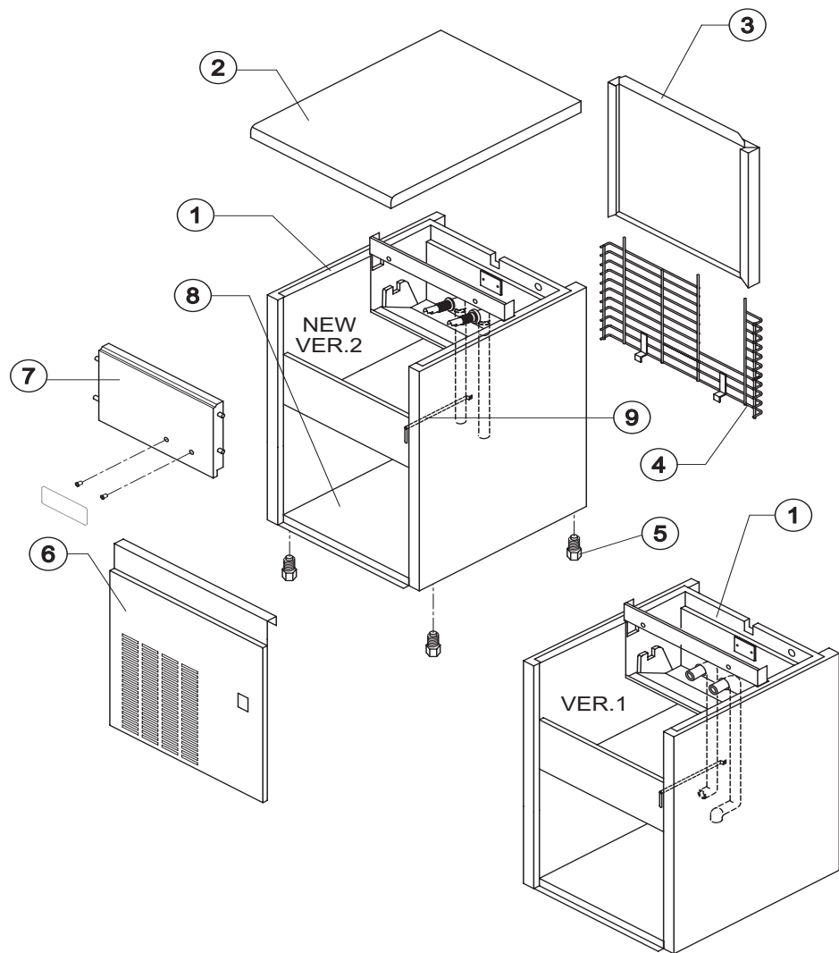
Ref. 1 - Assieme Mobile Schiumato/ Foamed Cabinet Assy Versione 1/Version 1
